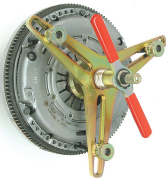
Fig. 3: Dispositivo de aperto com mandril de centragem
