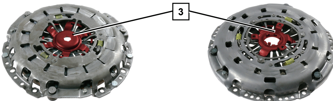
Fig. 5: Com peça de retenção (BMW)
