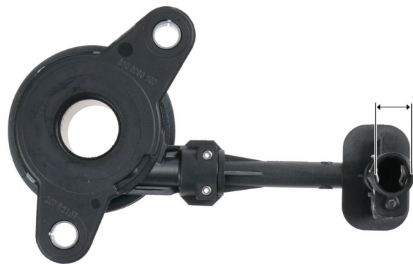
Fig. 4: CSC 3182 600 140 Durchmesser Hydraulikanschluss 12,2 mm
