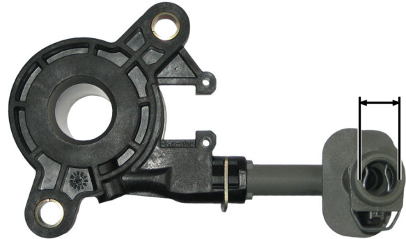
Fig. 2: CSC 3182 600 129 Durchmesser Hydraulikanschluss 13,3 mm
