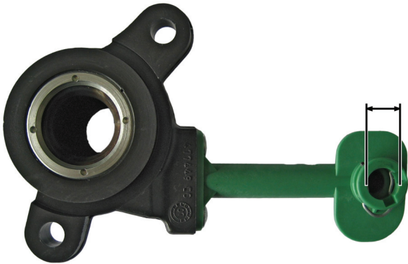
Fig. 1: CSC 3182 600 121 Durchmesser Hydraulikanschluss 11,7 mm
