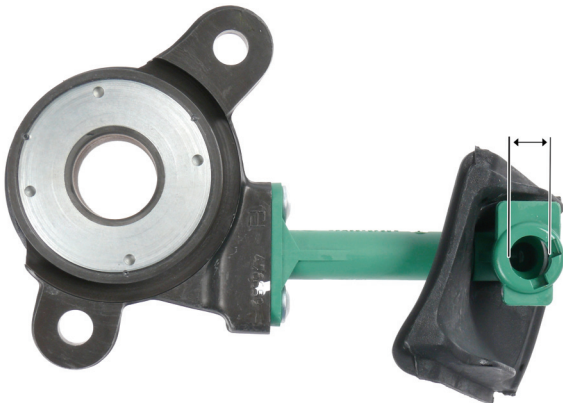
Fig. 3: CSC 3182 600 120 Durchmesser Hydraulikanschluss 12,2 mm
